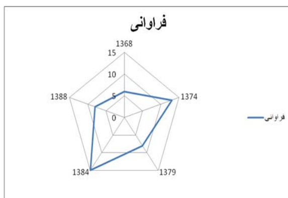
نمودار ۱- روند ظهور عبارت عمران روستایی در قوانین برنامه‌های توسعه
